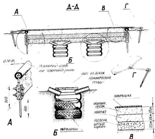
Рис. 7. Место для обучения приемам самостраховки, броскам, обезоруживаниям и болевым приемам: а — конструкция борта для укрепления ямы; б — устройство колодца для стока воды; в — конструкция наполнителя ямы; г — узел растяжки covers
