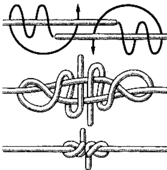
Рис. 34. Змеиный узел
