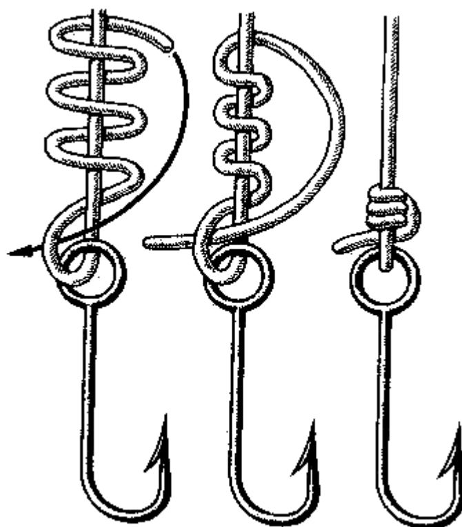
Рис. 126. Захватный узел
