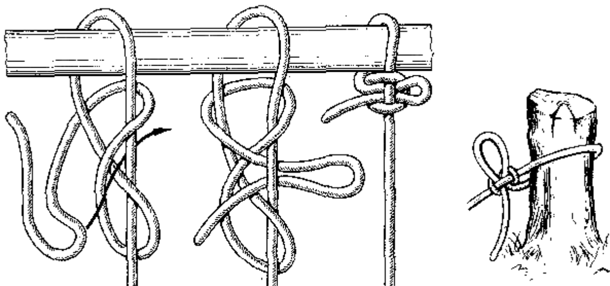
Рис. 102. Курьерский узел
