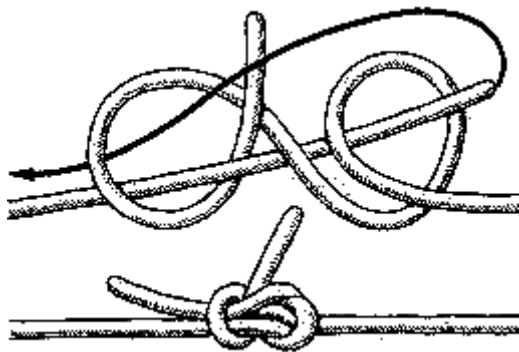
Рис. 37. Польский узел
