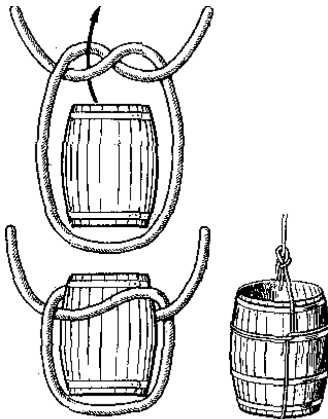
Рис. 108. Бочечный узел
