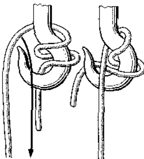
Рис. 106. Гачный узел со шлагом
