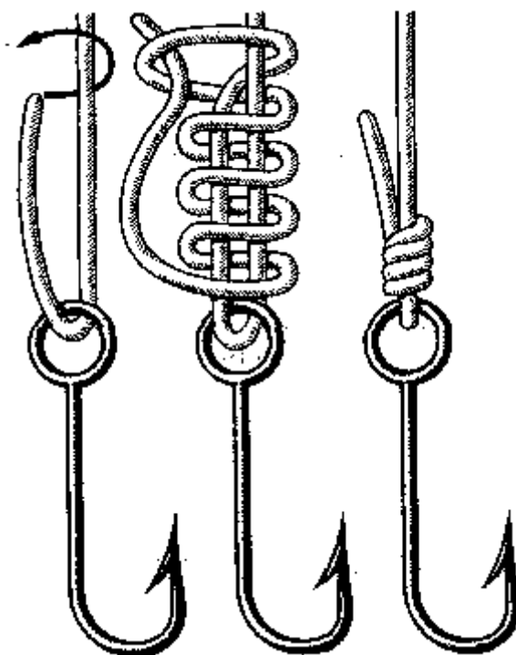
Рис. 127. Акулий узел
