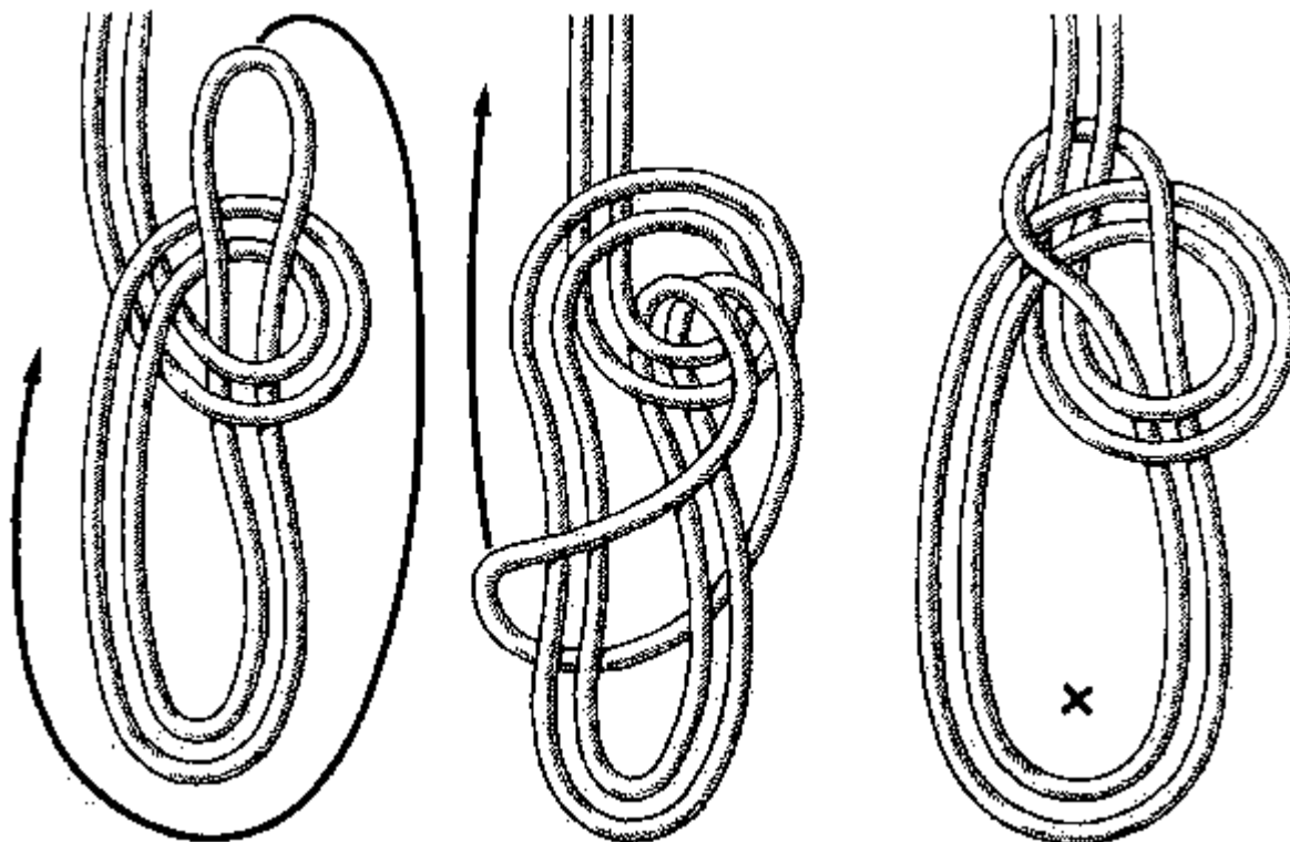
Рис. 77. Двойной беседочный узел
