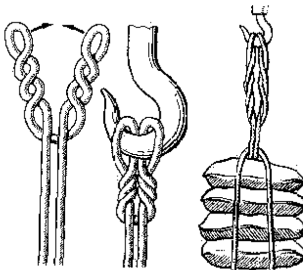
рис. 107. “Кошачья лапа”
