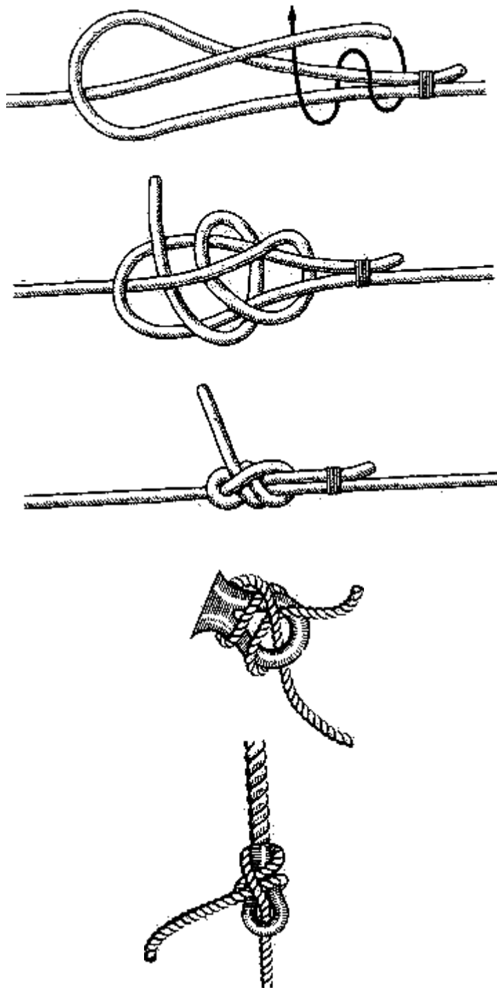
Рис. 39. Брам-шкотовый узел
