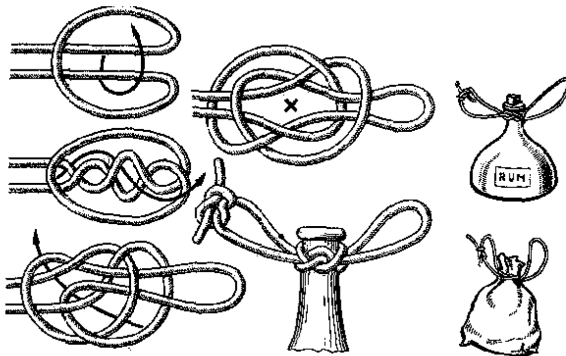
Рис. 111. Амфорный узел
