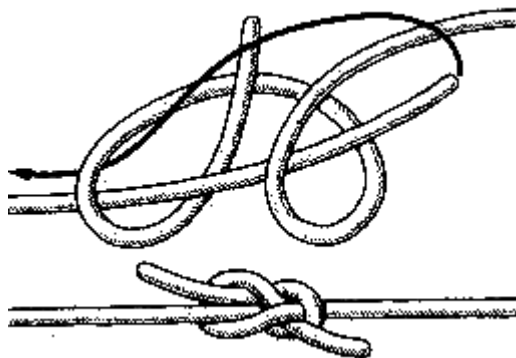
Рис. 36. Разносторонний узел
