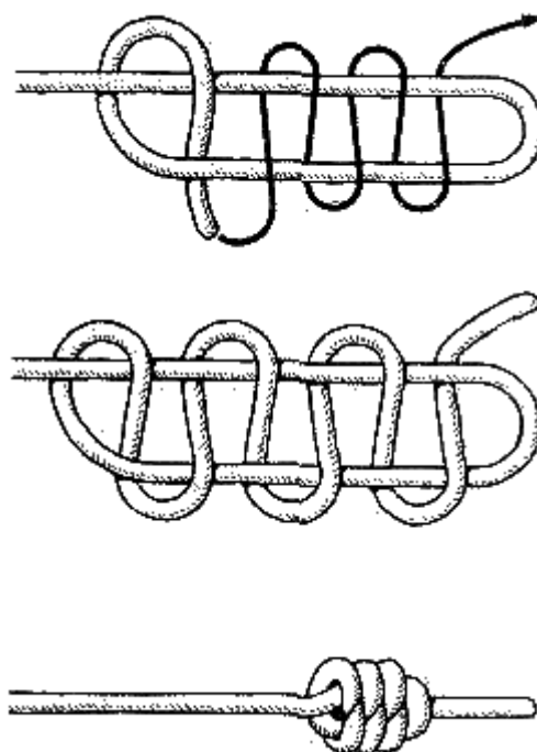
Рис. 7. Множественная восьмерка
