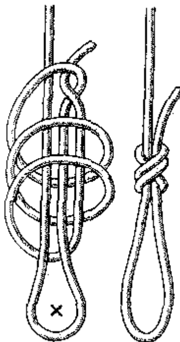
Рис. 87. Эшафотный узел
