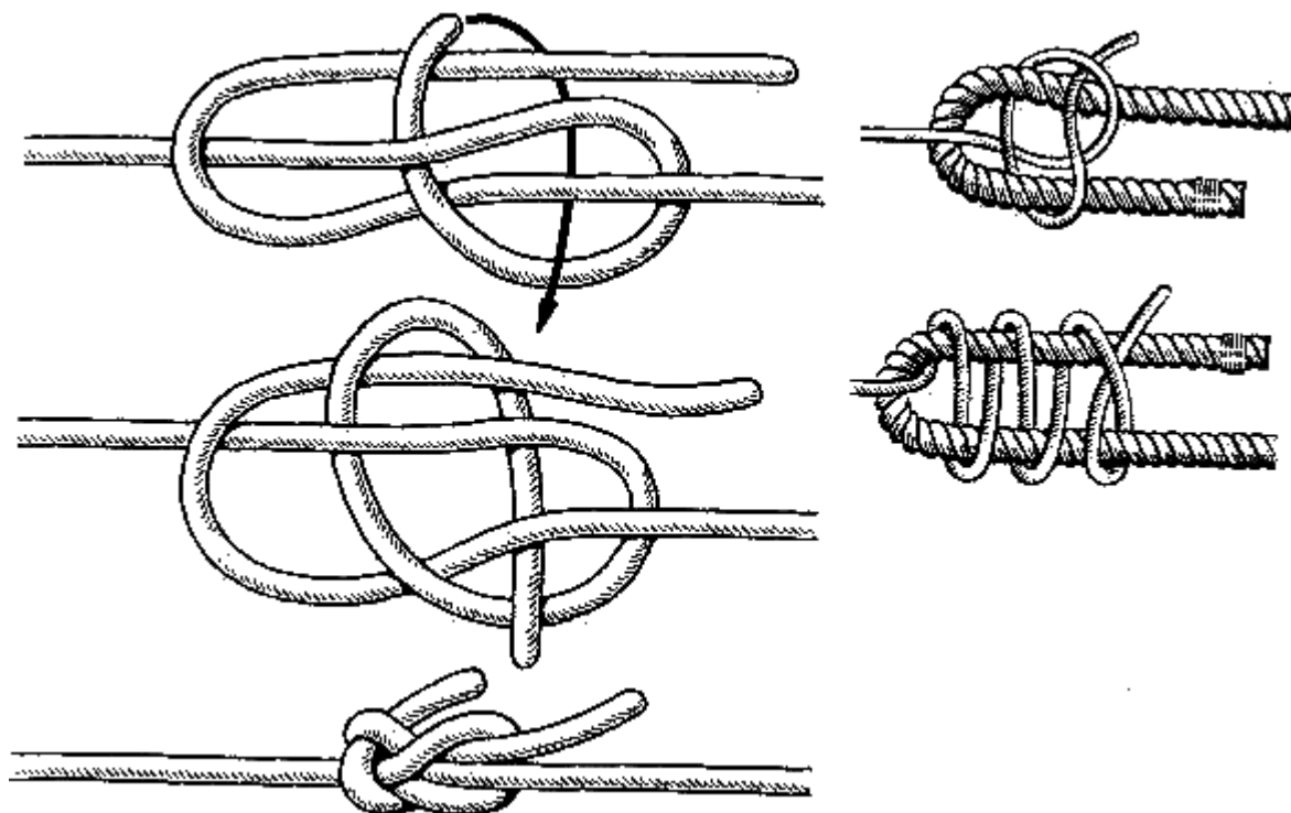
Рис. 40. Докерский узел (справа внизу – другой вариант узла)
