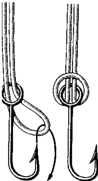
Рис. 119. Глухой узел
