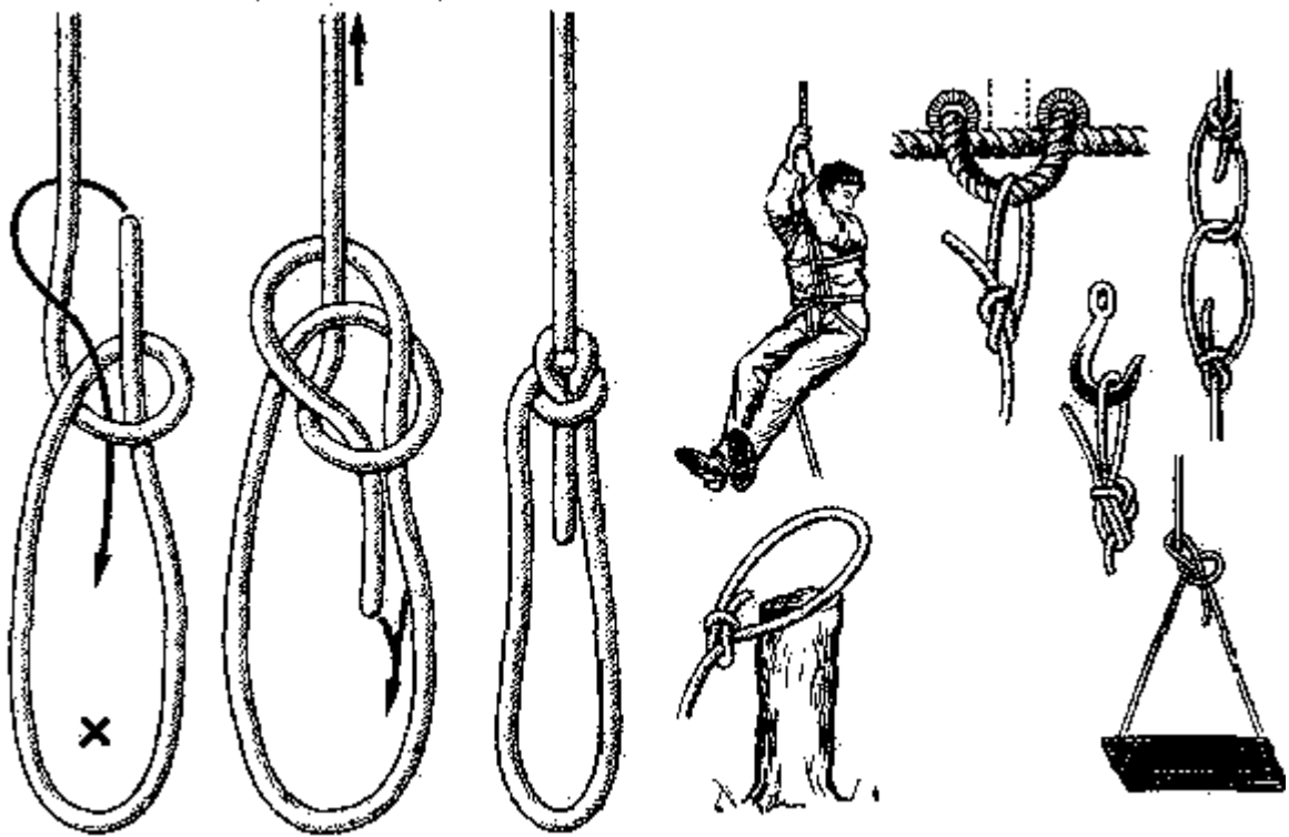
Рис. 76. Беседочной узел
