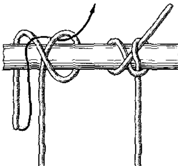
Рис. 54. Пикетный узел
