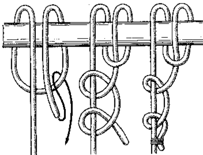
Рис. 16. Обратный штык
