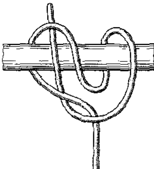
Рис. 53. Шахтерский узел
