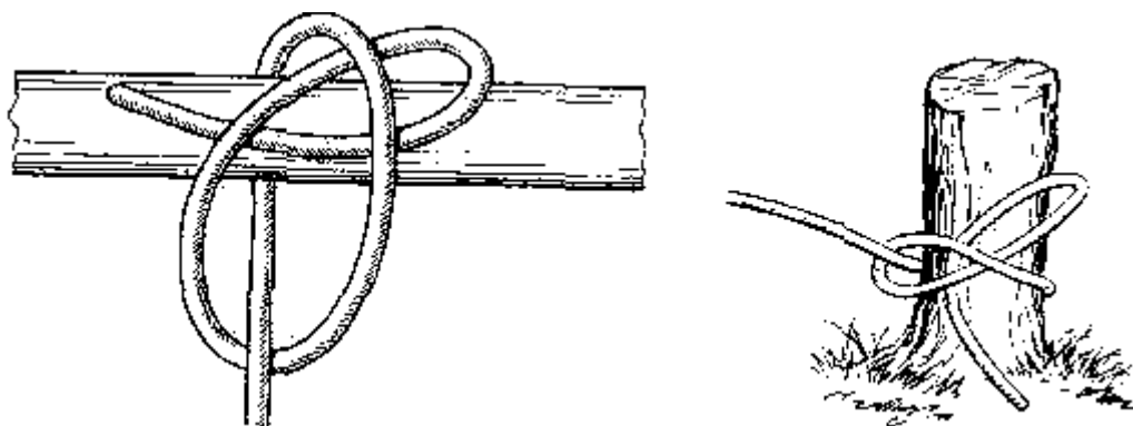
Рис. 98. Развязывающийся самозатягивающийся узел
