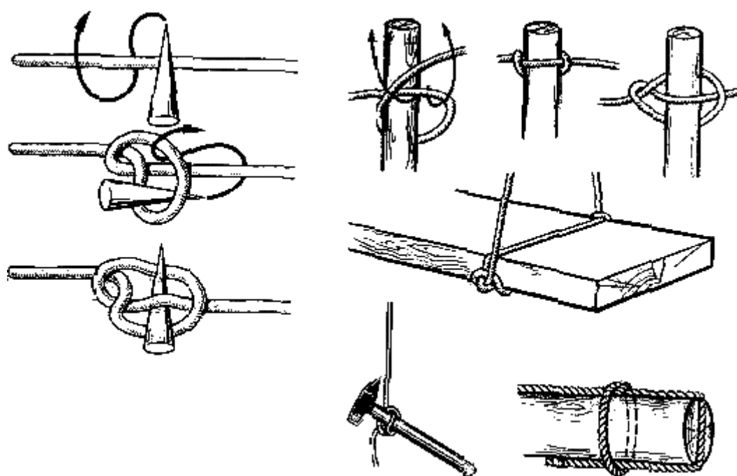
Рис. 110. Сваечный узел
