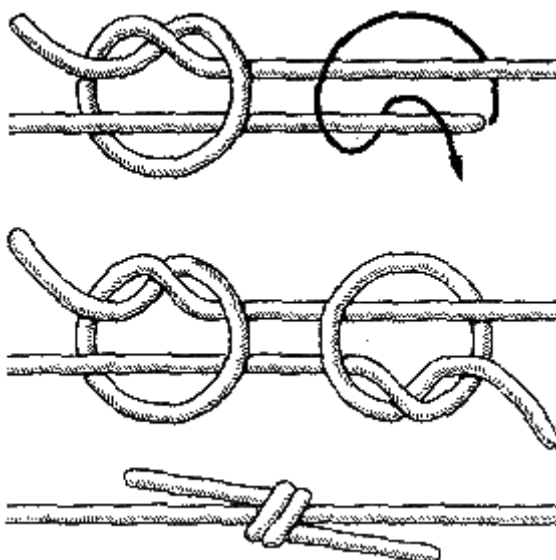
Рис. 33. Рыбацкий узел
