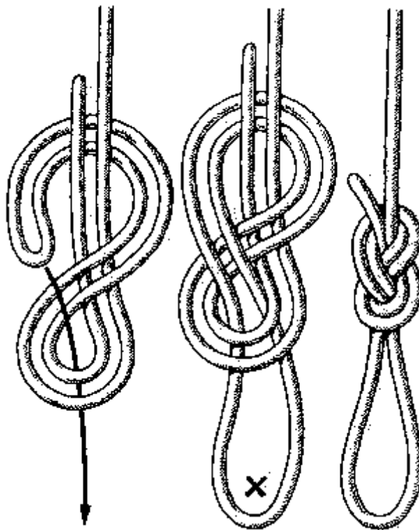
Рис. 68. Фламандская петля
