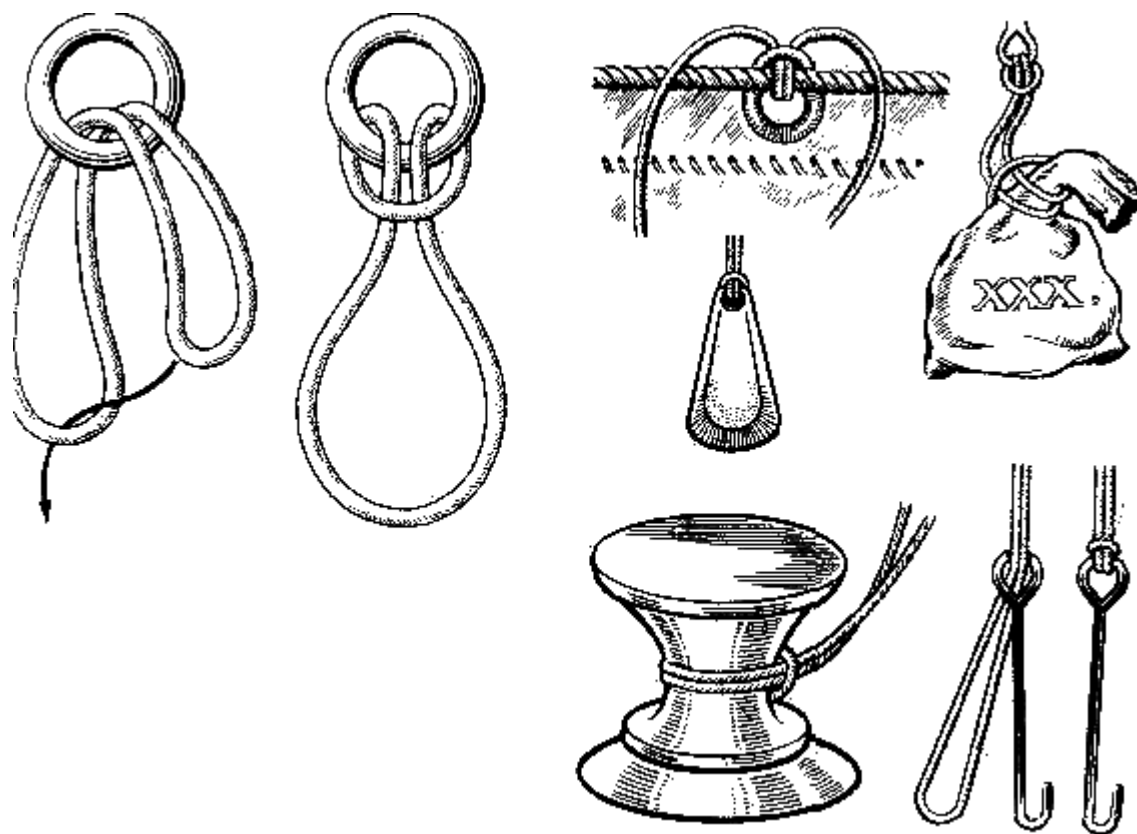
Рис. 47. Глухая петля
