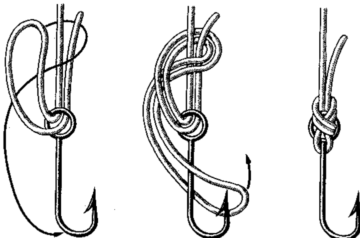
Рис. 124. Калифорнийский узел
