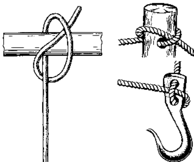
Рис. 44. Самозатягивающийся узел
