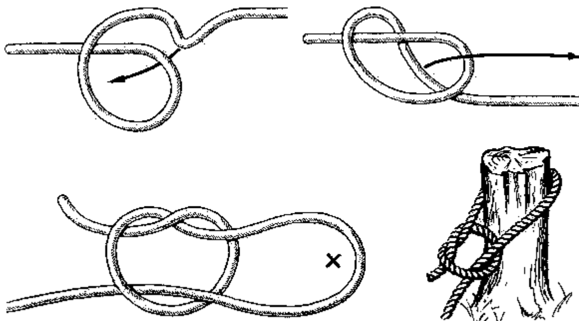
Рис. 82. Бегущий простой узел
