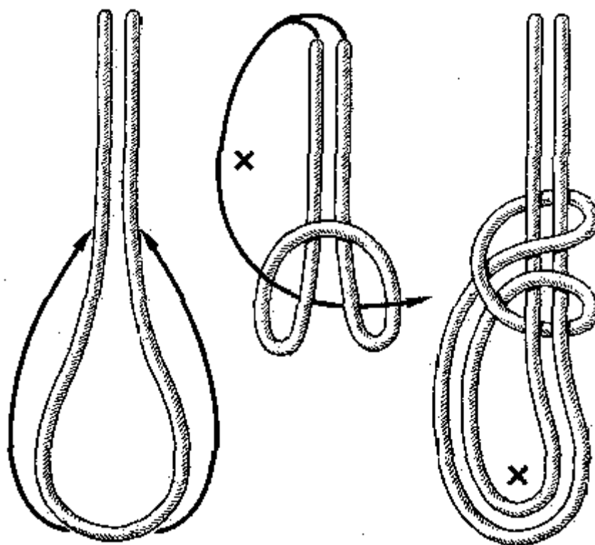
Рис. 84. Скользящая глухая петля
