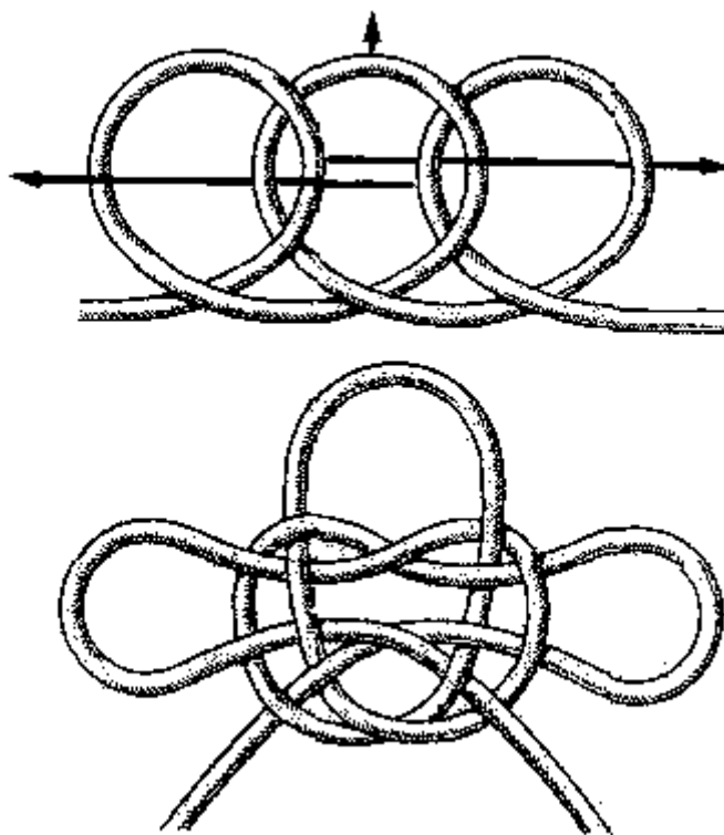
Рис.80. Топовый узел
