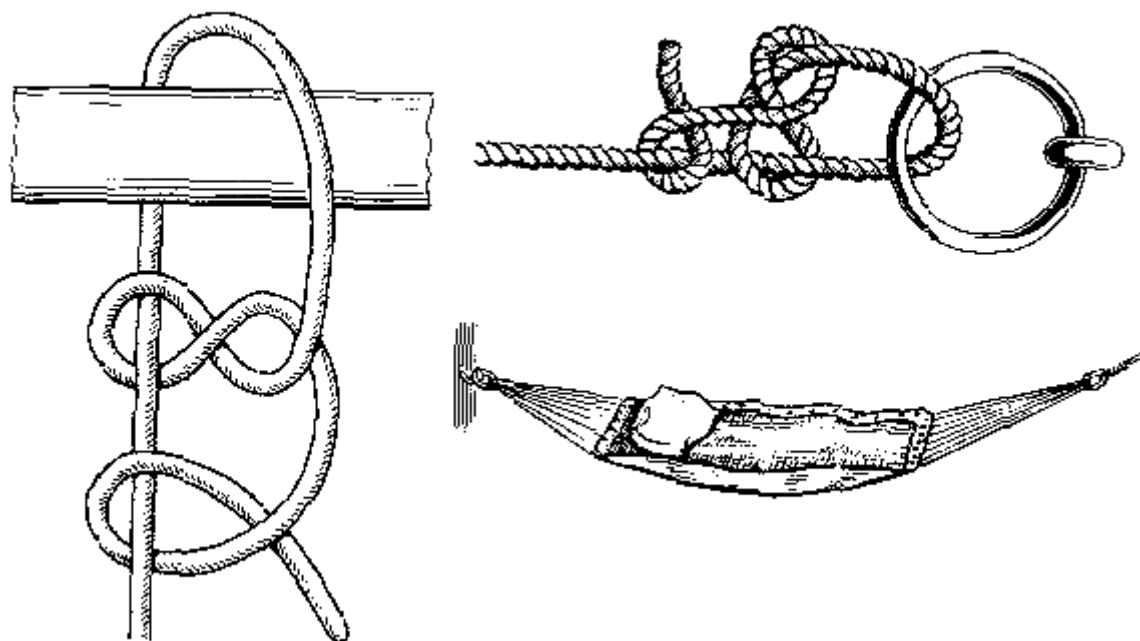
рис. 11. Кочный штык
