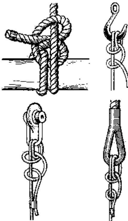
Рис. 15. Рыбацкий штык (якорный узел)
