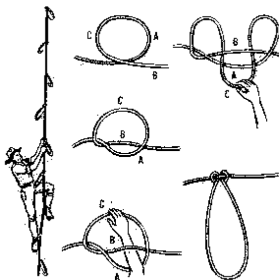
Рис. 73. Бурлацкая петля
