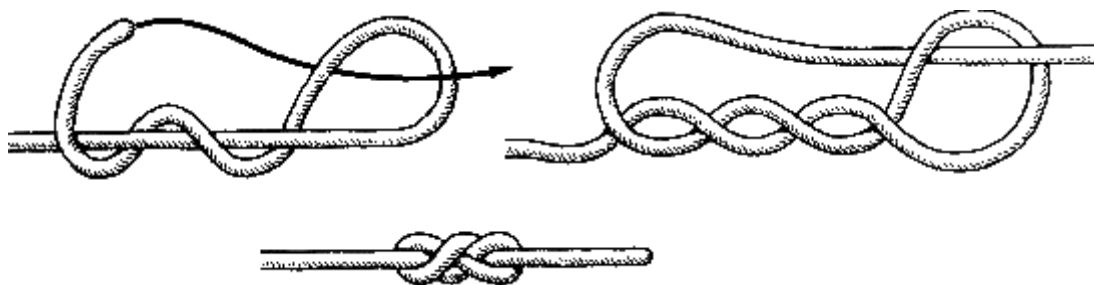
Рис. 4. Стивидорный узел
