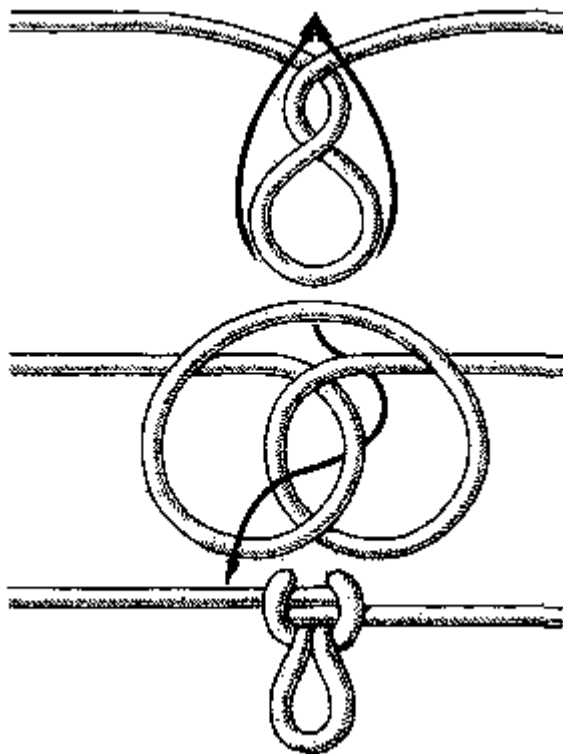
Рис. 74. Ездовая петля
