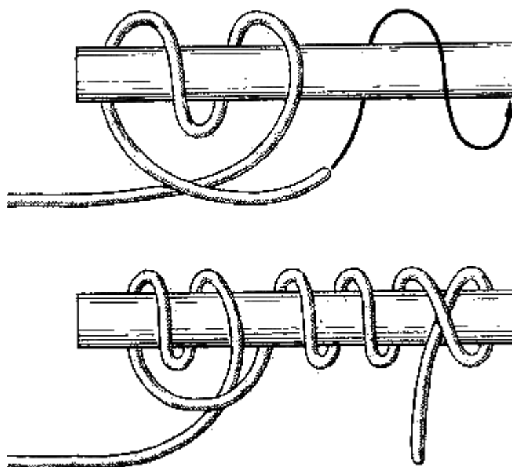
Рис. 60. Стопорный узел
