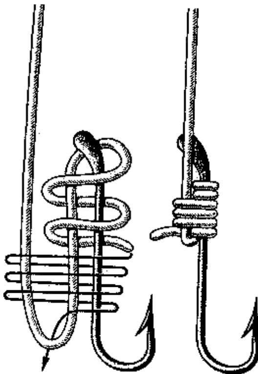
Рис. 125. Ступенчатый узел
