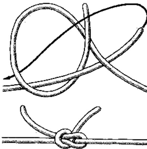
Рис. 35. Ткацкий узел
