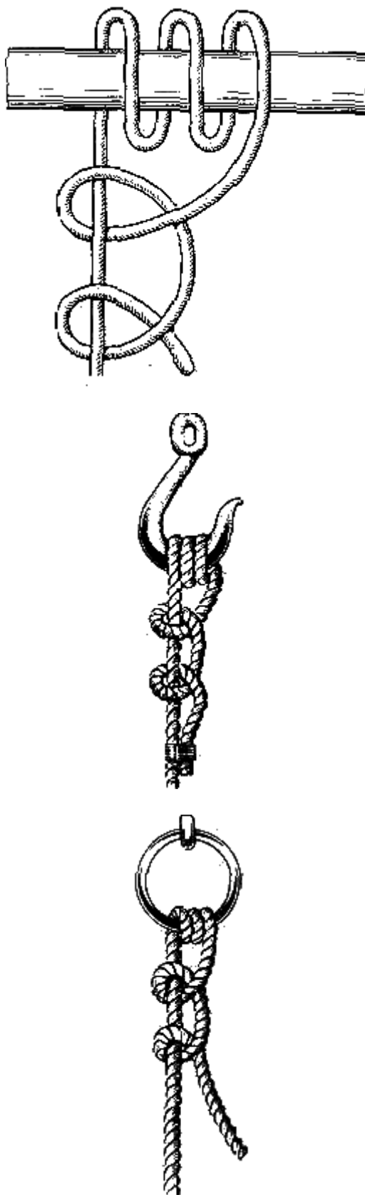
Рис. 13. Простой штык с двумя шлагами
