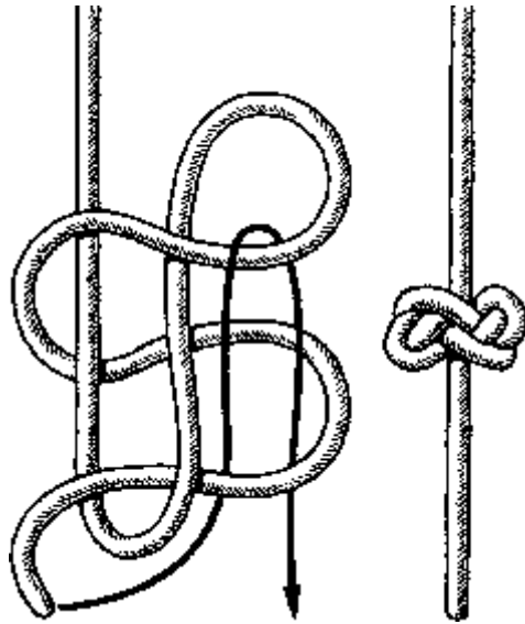
Рис. 137. Кордовый узел
