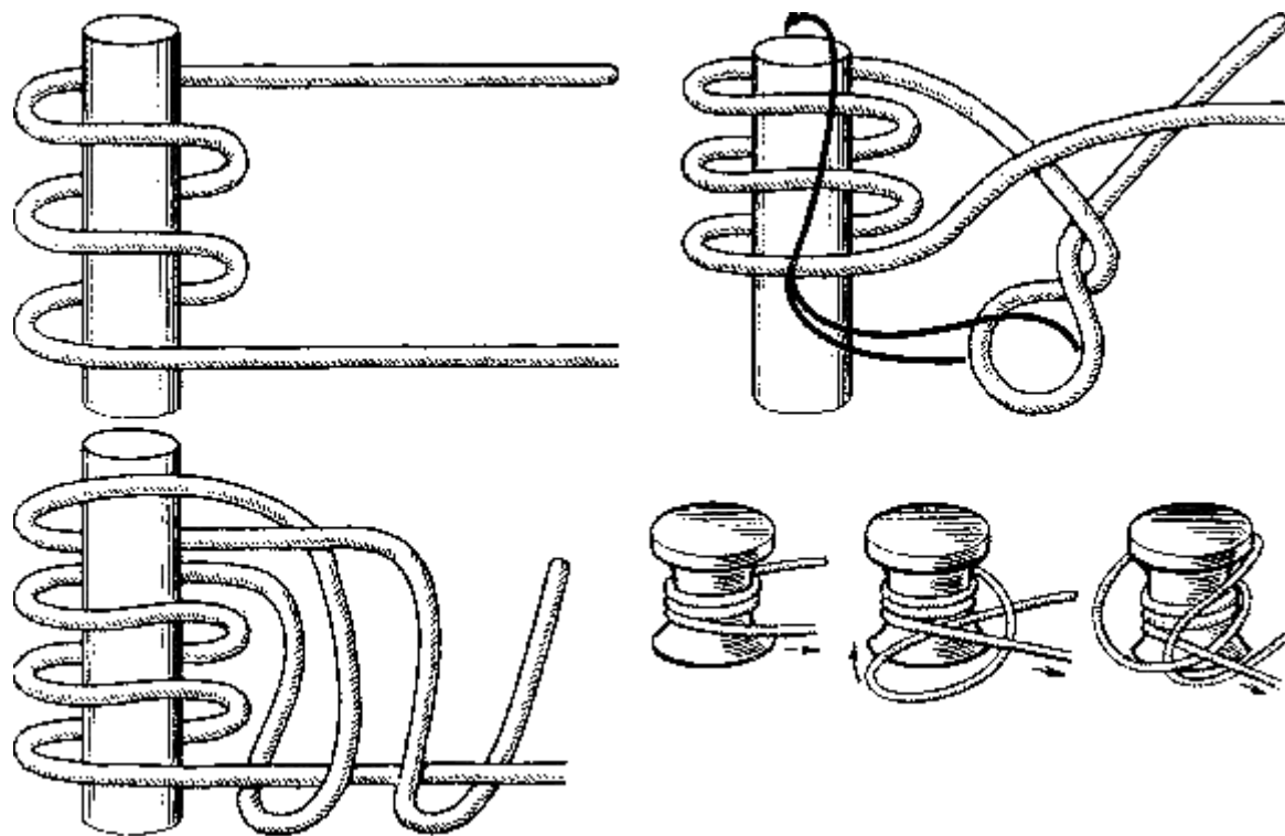
Рис. 19. Портовый узел
