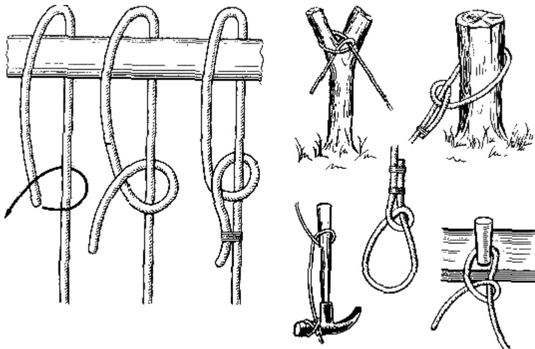
Рис. 9. Простой полуштык
