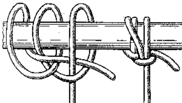
Рис. 58. Щучий узел
