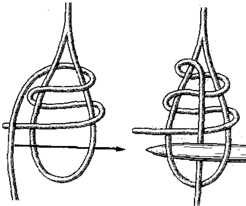
Рис. 112. Гинцевый узел
