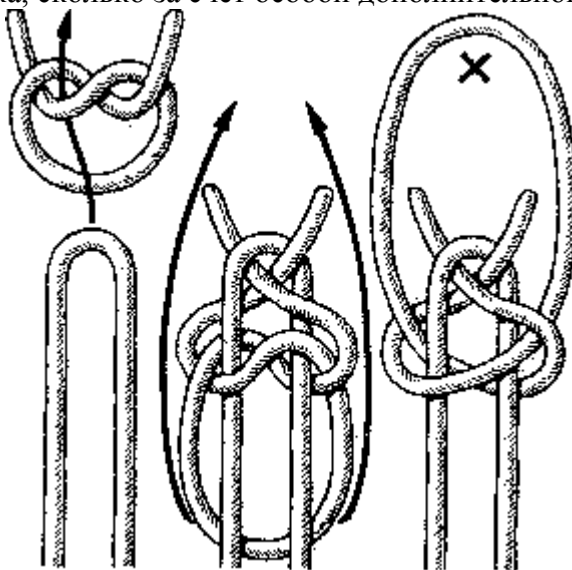
Рис. 116. Лучниковская петля
