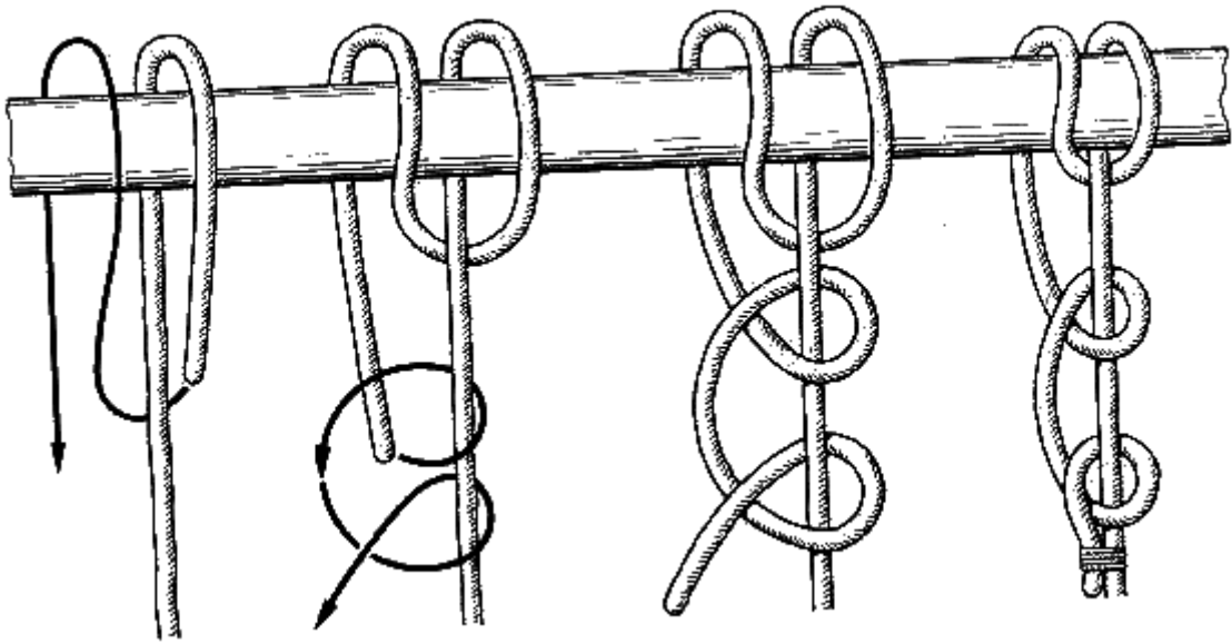
Рис. 14. Штык с обносом
