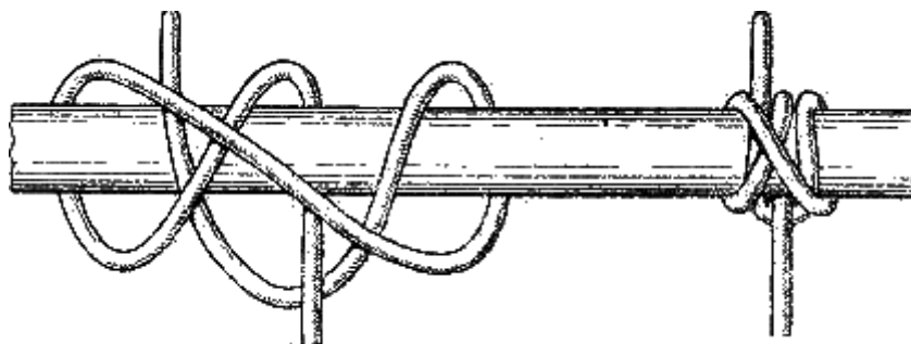
Рис. 61. Качельный узел
